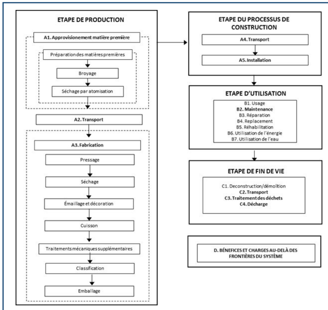
Figure 1. Diagramme avec les limites du système, les étapes et les processus pour la production d'1 m 2 de carreau céramique B1la 8,0 mm-8,8 mm.
