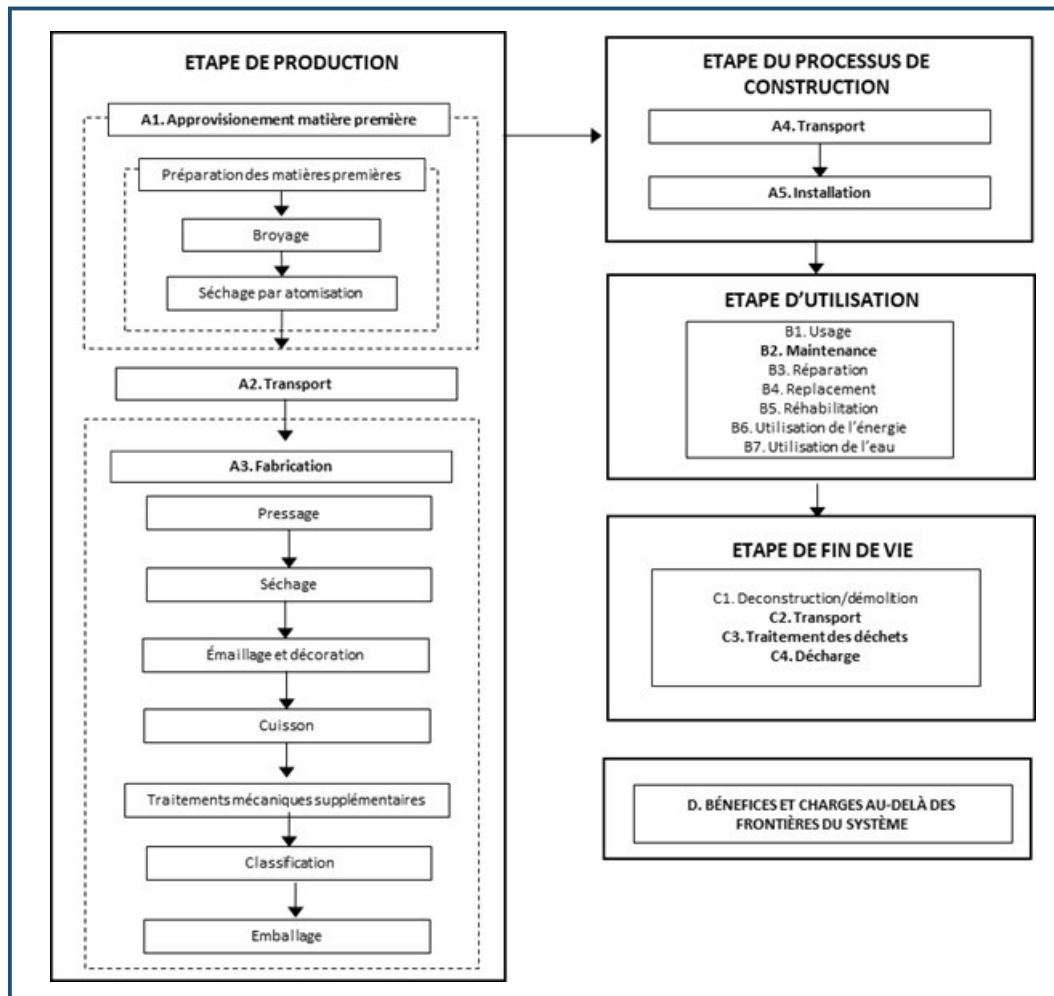
Figure 1. Diagramme avec les limites du système, les étapes et les processus pour la production d'1 m 2 de carreau céramique Bla 8,2 mm-10,8 mm.
